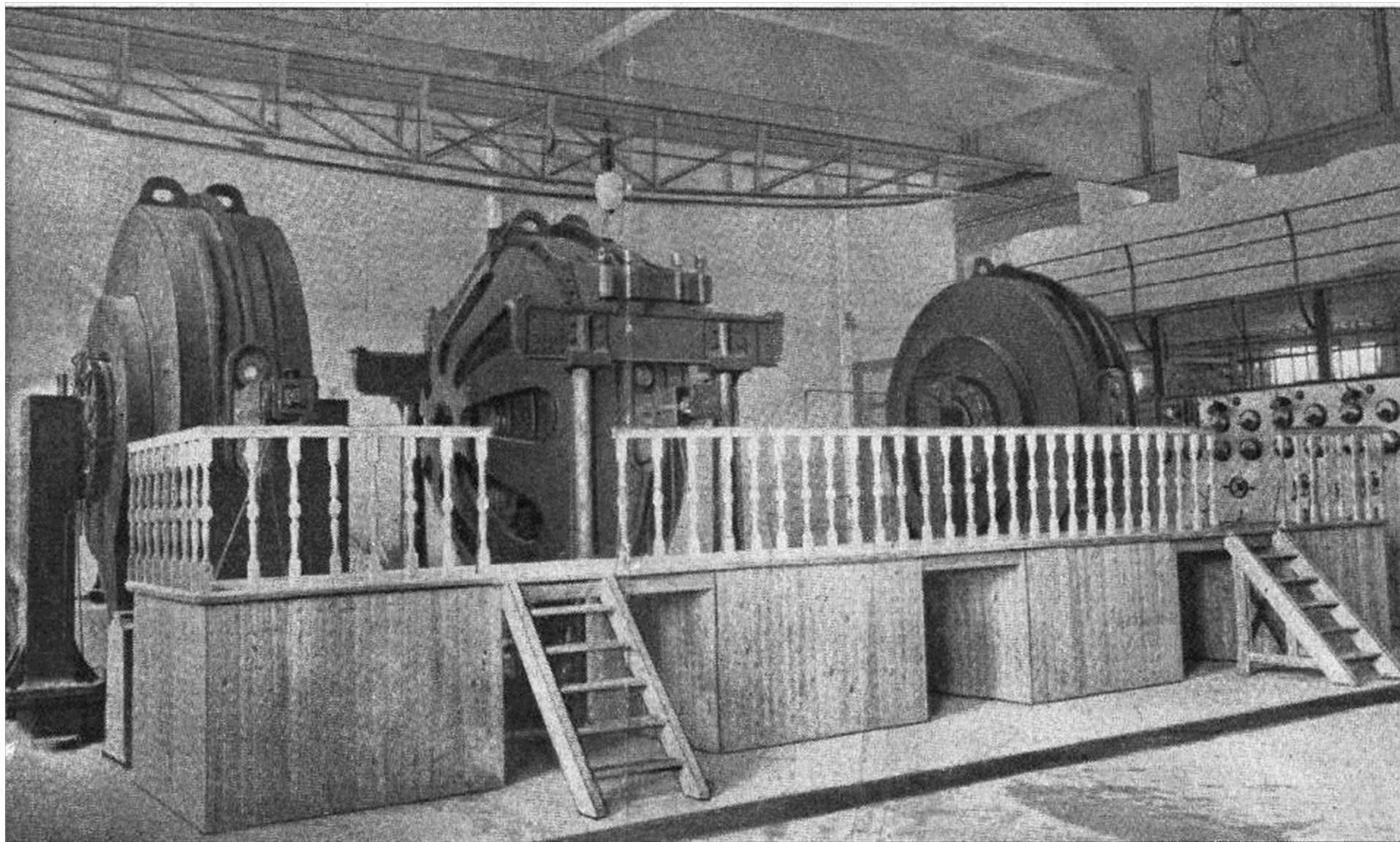
Birkeland-Eyde-ovner i forsøksfabrikken på Notodden – 1905
