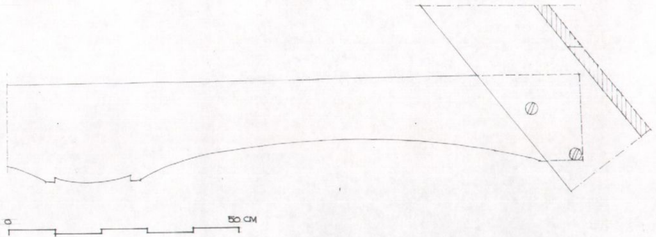
Detalj av østre sperrebind i skipets utvidelse mot vest, oppriss mot vest. OS 06
