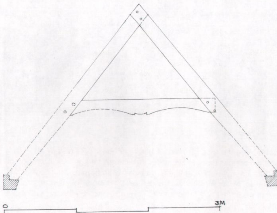
Østre sperrebind i skipets utvidelse mot vest, oppriss mot vest. OS 06
